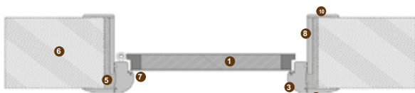
montaj usa + perv. 12x65 + contratoc + perv. 8x60
