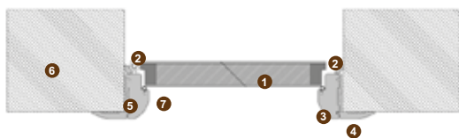
montaj usa + perv. 12x65 + bagheta toc
