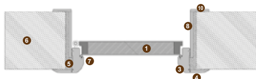
montaj usa + perv. 12x65 + contratoc + perv. 8x60
