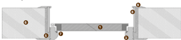
montaj usa + perv. 12x65 + contratoc + perv. 12x60
